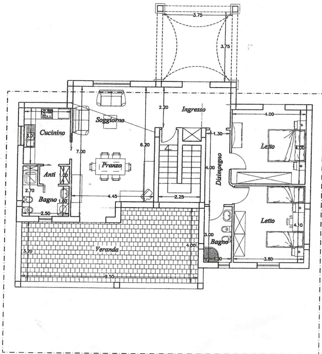
PIANTA PLANO TERRA
